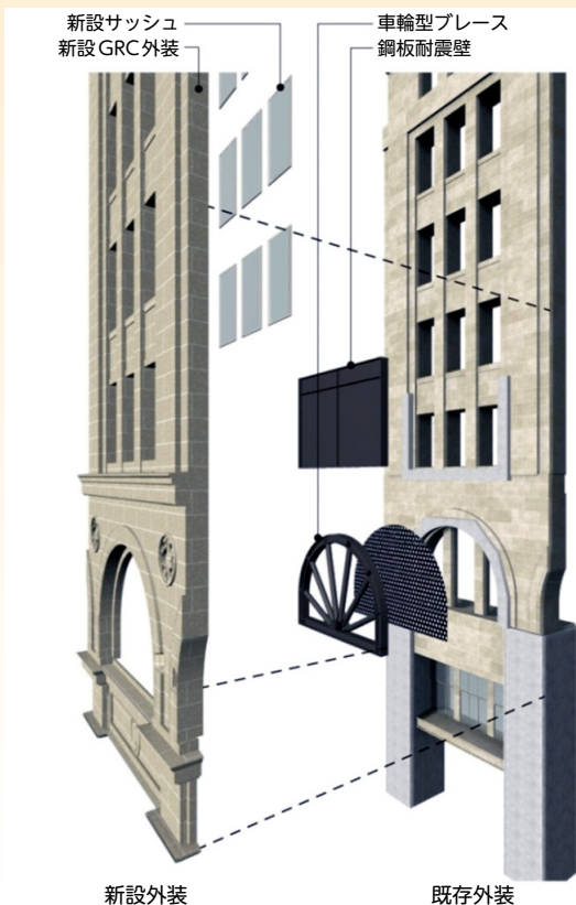
新設外装 既存外装 外装改修と耐震補強の概要
